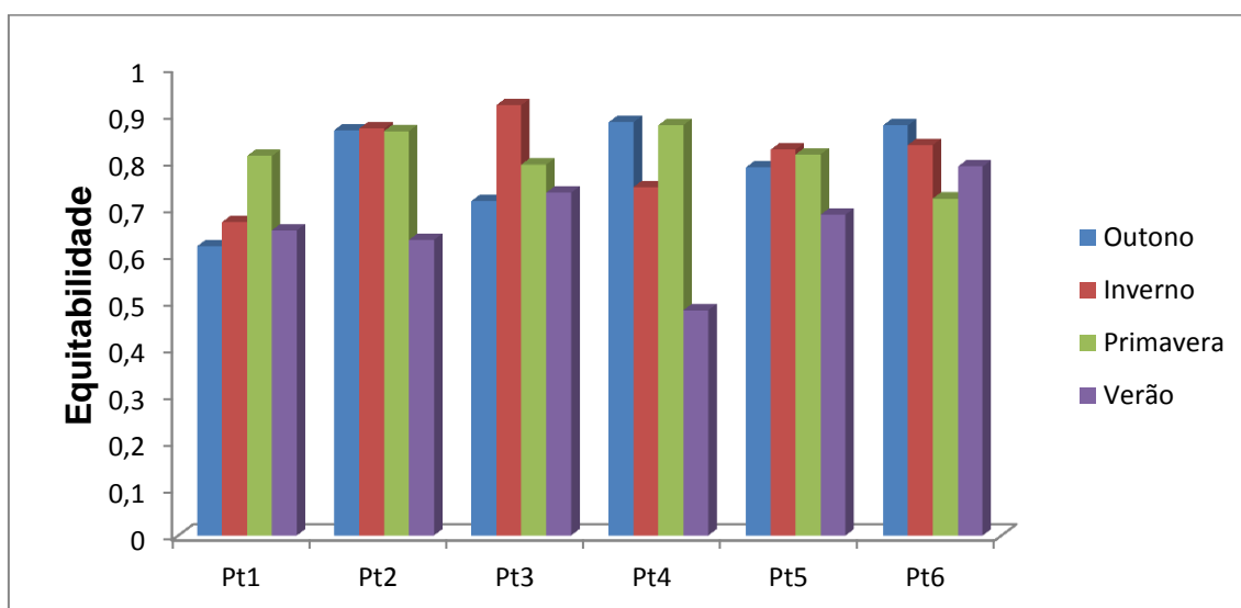
Figura 6. Valores da equitabilidade das espécies de peixes – pós-enchimento do reservatório da UHE Monjolinho. Os valores representam as médias entre as estações em cada ponto.
